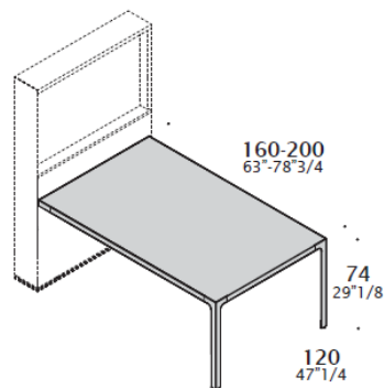
Tavolo. L160 + P120 + H74 L200 + P120 + H74
