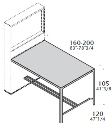
Tavolo. L160 + P120 + H105 L200 + P120 + H105
